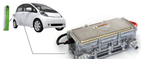
■ 電気自動車:空調用ヒータ部
